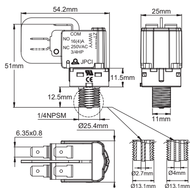
Filetage 1/4" NPSM
