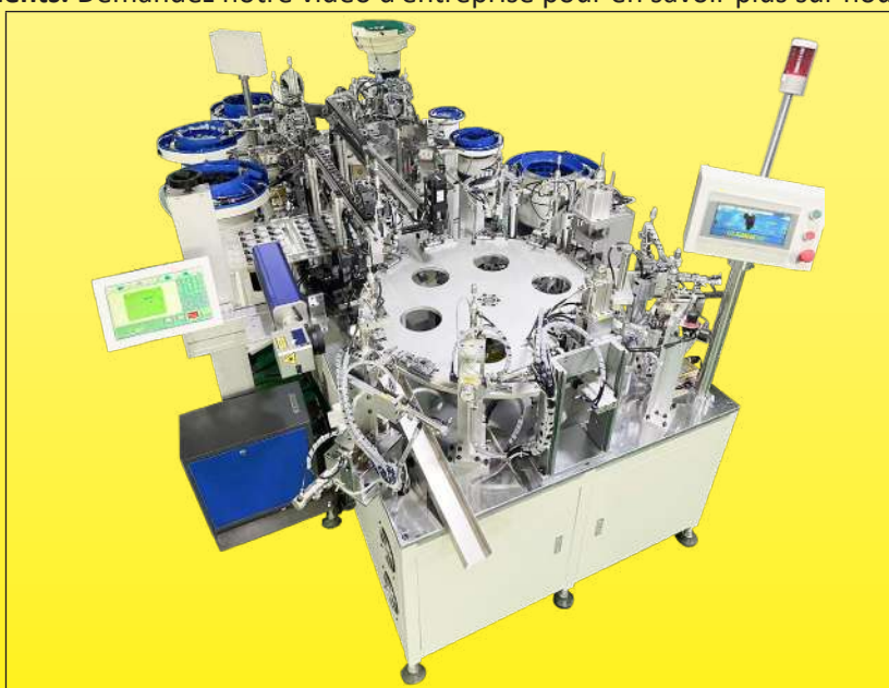
Ligne de fabrication totalement automatisée d'air switches et de pressostat (2022)
